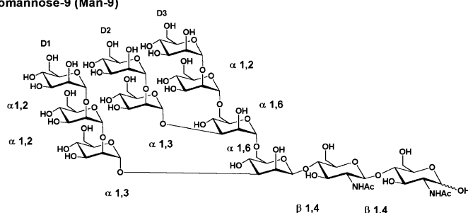
(4) Oligomannose-9 (Man-9)
