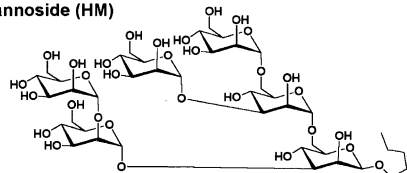
(3) Nonamannoside (NM)
