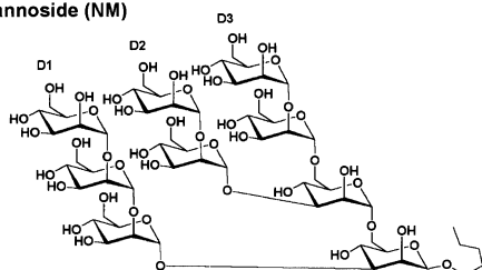
(4) Oligomannose-9 (Man-9)
